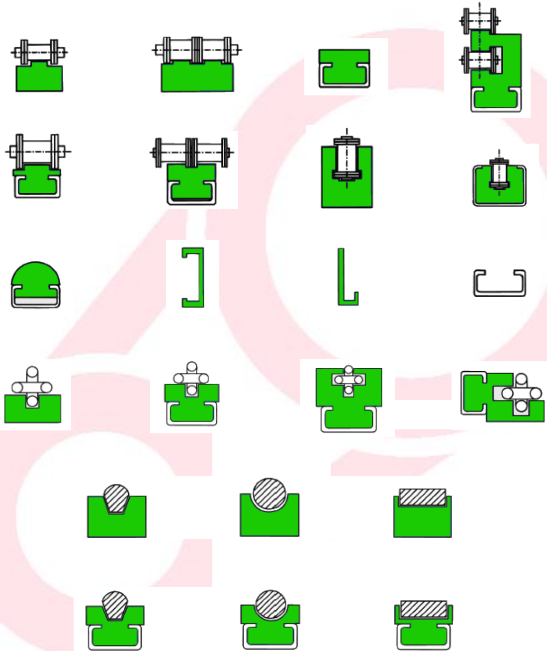
Geleideprofielen zijn verkrijgbaar in meerdere materialen en kwaliteiten
